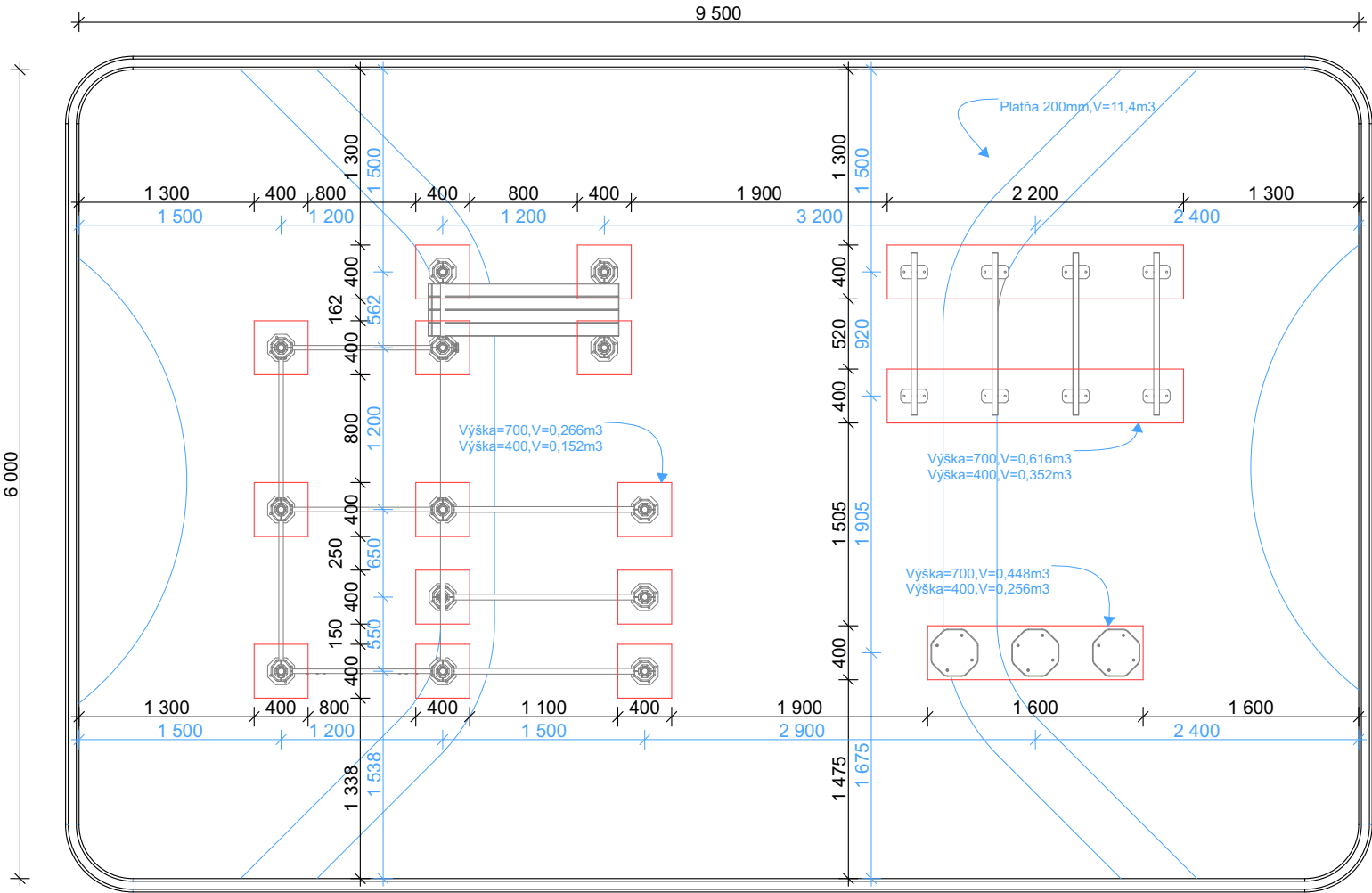
PÔDORYS:
